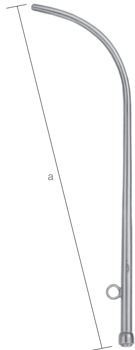
10317600 喉頭用吸引嘴管 九大型 a 180 外形 3.8
