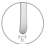
1030500 扁桃摘出刀 田所氏 全長210 a9 b7
