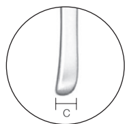
1030510 扁桃摘出刀 岡田氏 全長210 a15 b3 c7
